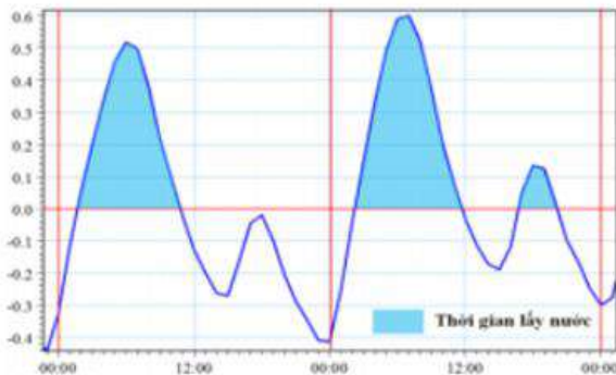
Hình 6: Sơ họa thời gian lấy nước cho mô hình
