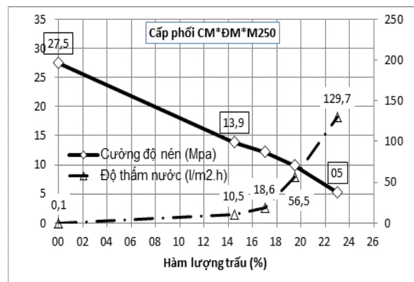
Hình 6: Ảnh hưởng hàm lượng trấu tới cường độ và độ thấm nước của bê tông khi sử dụng cát M=2,13 + đá mi
