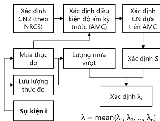
Hình 4: Quy trình xác định λ của lưu vực
