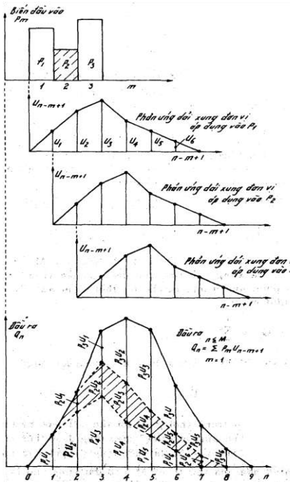
Hình 5: Nguyên tắc xếp chồng đường
