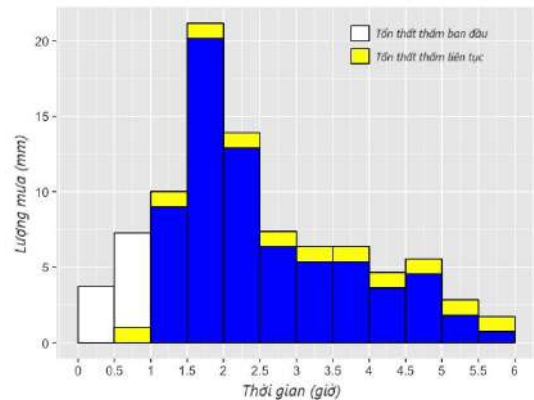
Hình 2: Minh họa tổn thất thấm ban đầu ( I_a ) và tổn thất thấm liên tục ( F_a )
