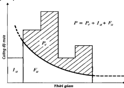
Hình 1: Các biến số của tổn thất dòng chảy trong phương pháp SCS:
