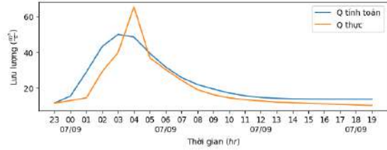
Hình 8: Kết quả mô phỏng lũ cho trận lũ ngày 21/8/2022 và trận lũ 07/9/2023
