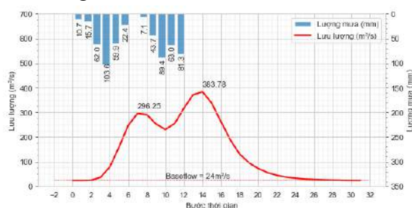
Hình 3: Dữ liệu của một trận lũ của một lưu vực
