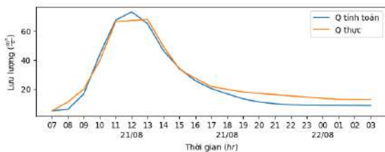
Hình 7: Kết quả xây dựng đường quá trình lưu lượng đơn vị lưu vực suối Bắc Cường
