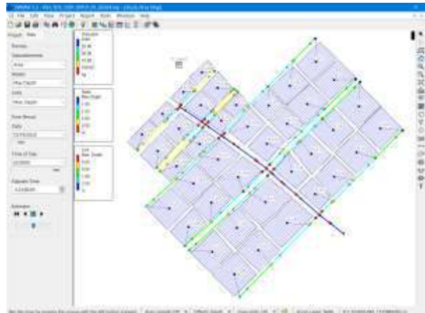
Hình 3: Kết quả thiết lập hệ thống tiêu thoát nước cho khu vực dự án
