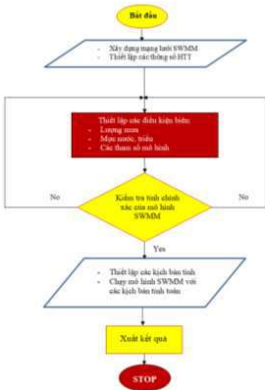
Hình 2: Sơ đồ khối tính toán dòng chảy cho hệ thống tiêu thoát nước trong KCN
