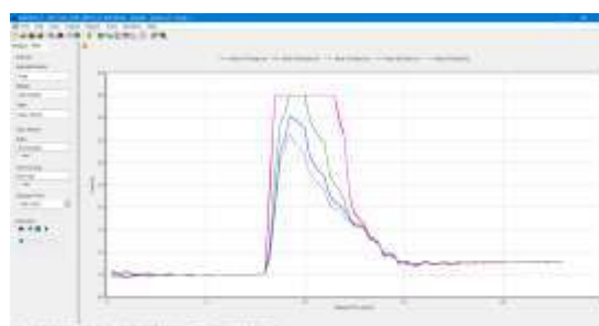
Hình 6: Quá trình MN tại tuyến cống 1 KCN với các điểm G1-2-3-17-18 (các tiểu vùng 2-17-18 bị úng ngập do chảy tràn bề mặt)
