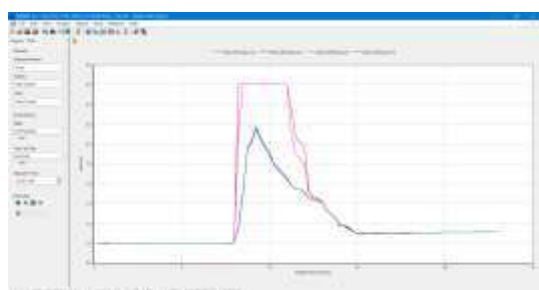
Hình 5: Quá trình MN tại tuyến cống 1 khu TĐC với các điểm G29-30-35-36 (các tiểu vùng 29-35 bị úng ngập do chảy tràn bề mặt)
