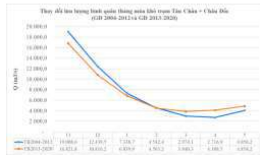
Hình 8: Thay đổi lưu lượng trung bình tháng mùa khô giai đoạn 2004-2012 và 2013-2020
