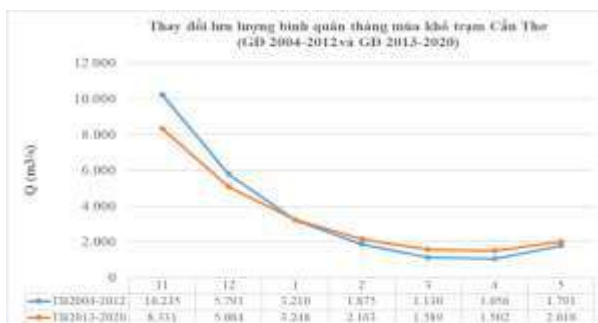
Hình 15: Thay đổi lưu lượng trung bình tháng mùa khô trạm Cần Thơ giai đoạn 2004-2012 và 2013-2020
