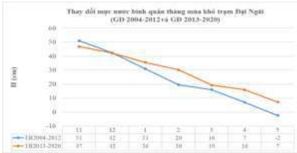
Hình 16: Thay đổi mực nước lớn nhất mùa khô trạm Đại Ngãi giai đoạn 2004-2012 và 2013-2020
