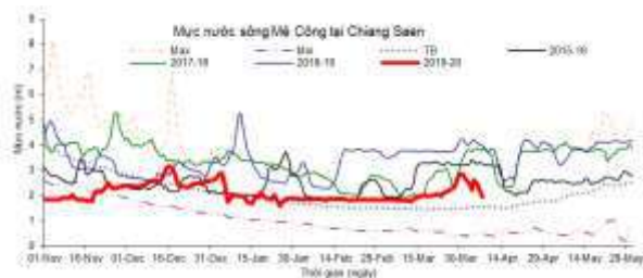
Hình 5: Diễn biến mực nước mùa kiệt trạm Chiang Saen
