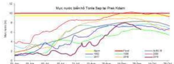
Hình 3: Diễn biến mực nước biển hồ Tonle Sap
