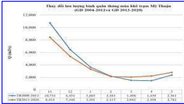
Hình 10: Thay đổi lưu lượng trung bình tháng mùa khô trạm Mỹ Thuận giai đoạn 2004-2012 và 2013-2020
