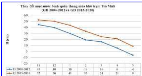
Hình 11: Thay đổi mực nước lớn nhất mùa khô trạm Trà Vinh giai đoạn 2004-2012 và 2013-2020
