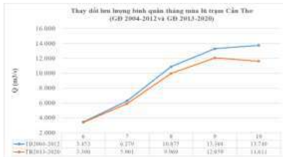
Hình 14: Thay đổi lưu lượng trung bình tháng mùa lũ trạm Cần Thơ giai đoạn 2004-2012 và 2013-2020
