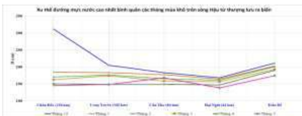
Hình 18: Xu thế đường mực nước cao nhất mùa khô trên sông Hậu từ thượng lưu ra biển
