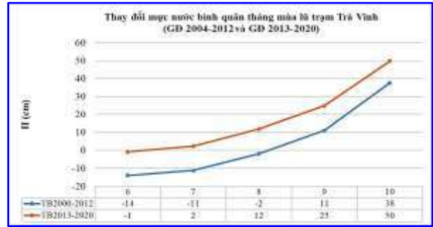
Hình 12: Thay đổi mực nước lớn nhất mùa lũ trạm Trà Vinh giai đoạn 2004-2012 và 2013-2020
