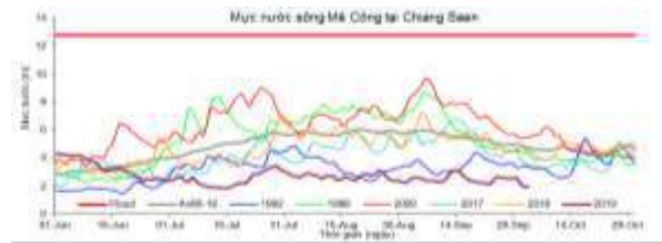
Hình 1: Diễn biến mực nước lũ trạm Chiang Saen
