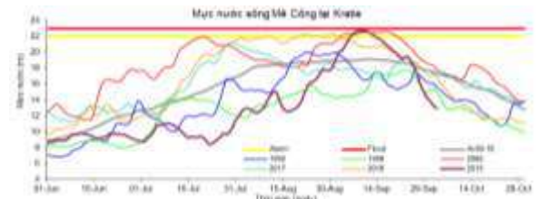
Hình 2: Diễn biến mực nước lũ trạm Kratie
