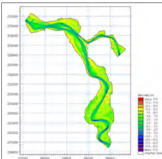
Hình 4: Thiết lập địa hình mô hình 2D sông Hồng đoạn qua Hà Nội
