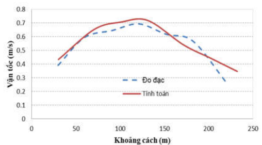
Hình 6: Kết quả kiểm định sự tương tự về trường phân bố Vtb thủy lực trên MC ngang lúc 17 h ngày 17/6/2018 tại 2 MC trên sông Hồng khu vực Hà Nội
