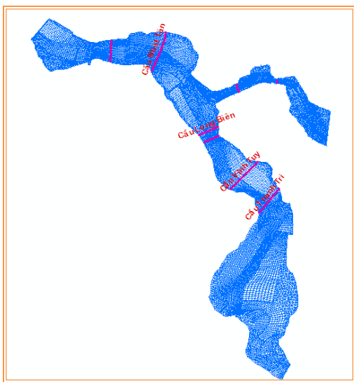
Hình 3: Thiết lập lưới tính toán tổng thể cho mô hình 2D sông Hồng đoạn qua Hà Nội
