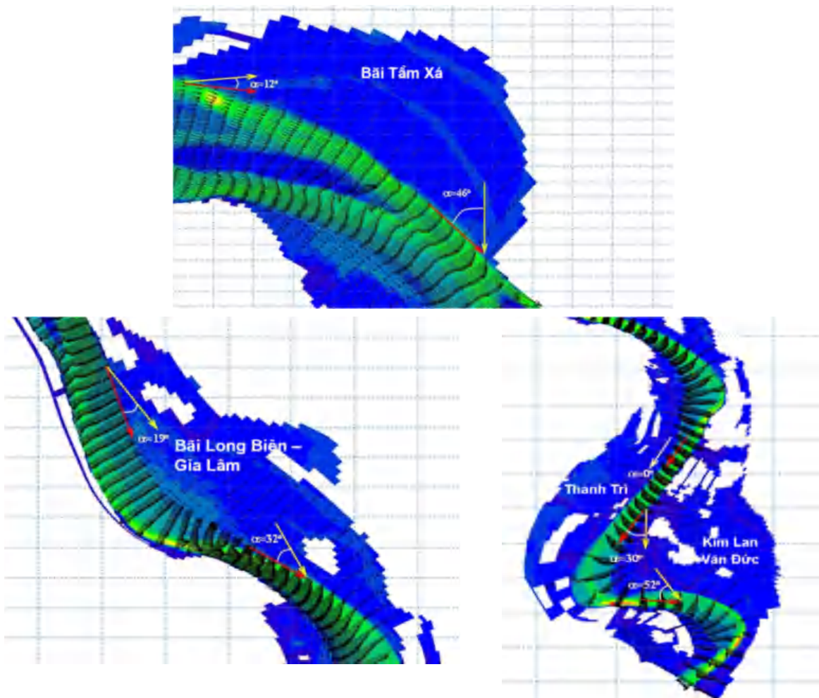
Hình 9: Góc ( \alpha ) thể hiện sự tương tác dòng chảy lũ giữa lòng và bãi sông trên các khu vực thuộc đoạn sông Hồng qua Hà Nội [4]
