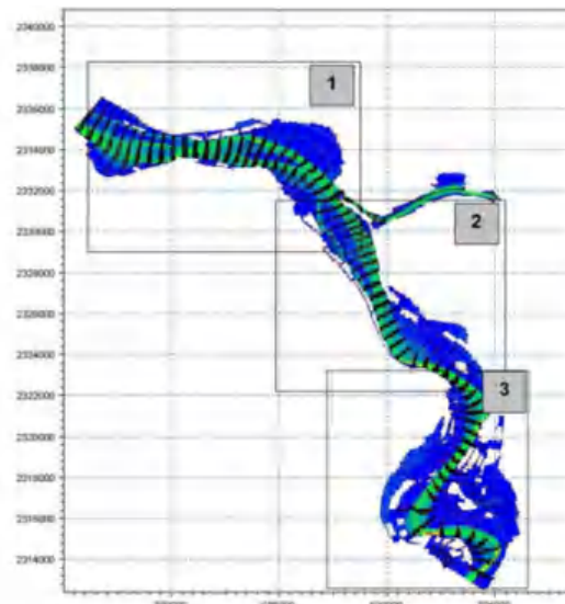
Hình 7: Trường phân bố vận tốc dòng chảy trên các mặt cắt ngang đoạn sông Hồng qua Hà Nội, với lũ thiết kế (lũ 300 năm)
