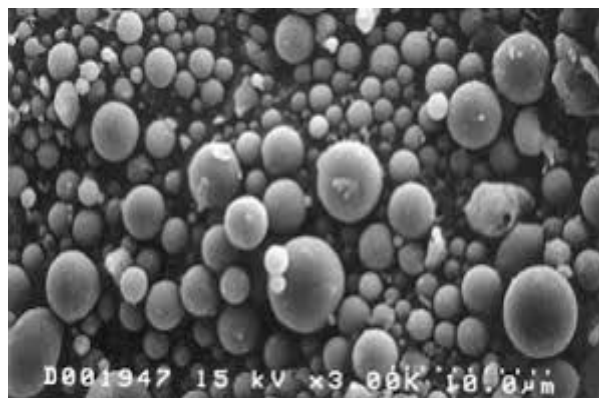
Hình 2.1: Hình dạng hạt tro bay ở trạng thái tự nhiên và qua kính hiển vi điện tử quét
