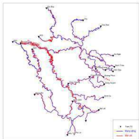
Hình 2: Phạm vi mô hình thủy lực 1 chiều
