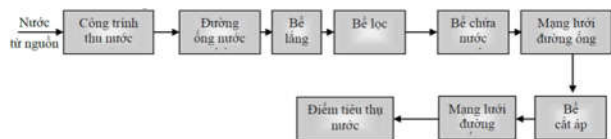
Hình 7: Quy trình công nghệ cấp nước tự chảy sử dụng nước từ khe suối [6]
