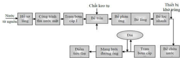
Hình 6: Quy trình công nghệ cấp nước tự chảy sử dụng nước sông [9]
