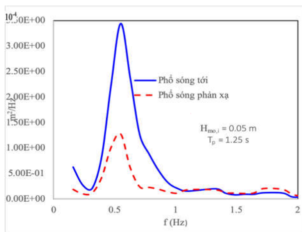
Hình 7: Biến đổi phổ sóng tới và sóng phản xạ trong quan trắc mô hình vật lý
