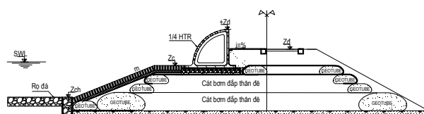
Hình 1: Mặt cắt đê biển có kết cấu tiêu sóng hình trụ rỗng trên đỉnh
