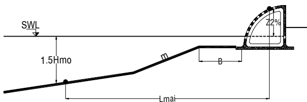
Hình 4: Xác định góc nghiêng mái dốc trung bình (TAW 2002)
