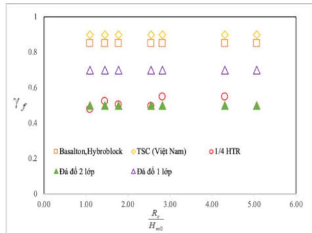
Hình 6: Quan hệ độ lưu không tương đối và hệ số chiết giảm sóng tràn
