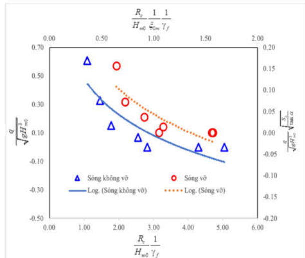
Hình 5: Sóng tràn qua đê có 1/4HTR tại đỉnh, sóng vỡ và không vỡ ứng với chu kỳ T_{m-1,0}
