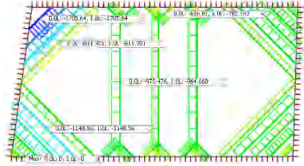
b) Lực dọc thanh chống
