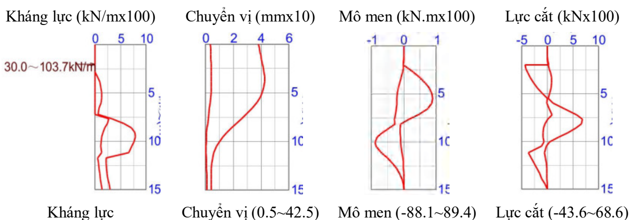
Hình 10: Chuyển vị và nội lực của tường
