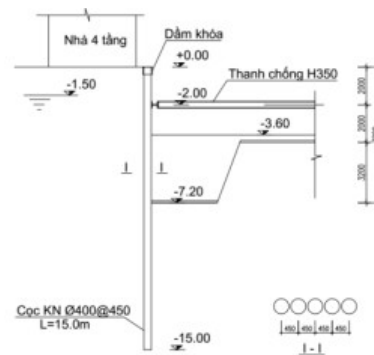
Hình 3: Mặt cắt ngang hố móng
