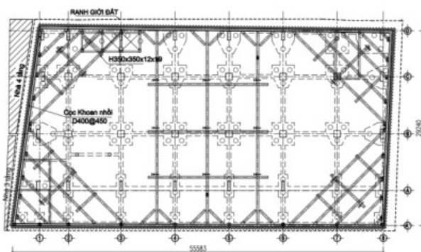
Hình 2: Mặt bằng hồ móng
