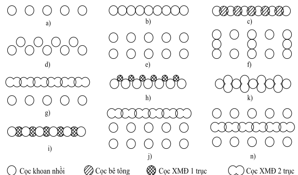
Hình 1: Hình thức bố trí tường cọc khoan nhồi kết hợp cọc bê tông cốt thép hoặc cọc xi măng đất
