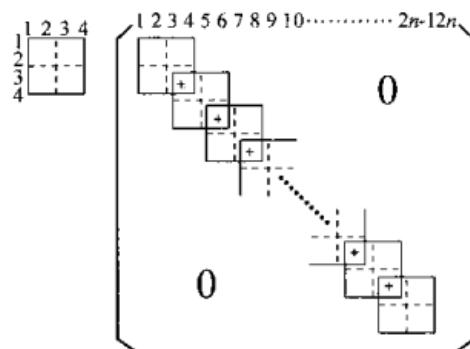
Hình 7: Ma trận độ cứng K
