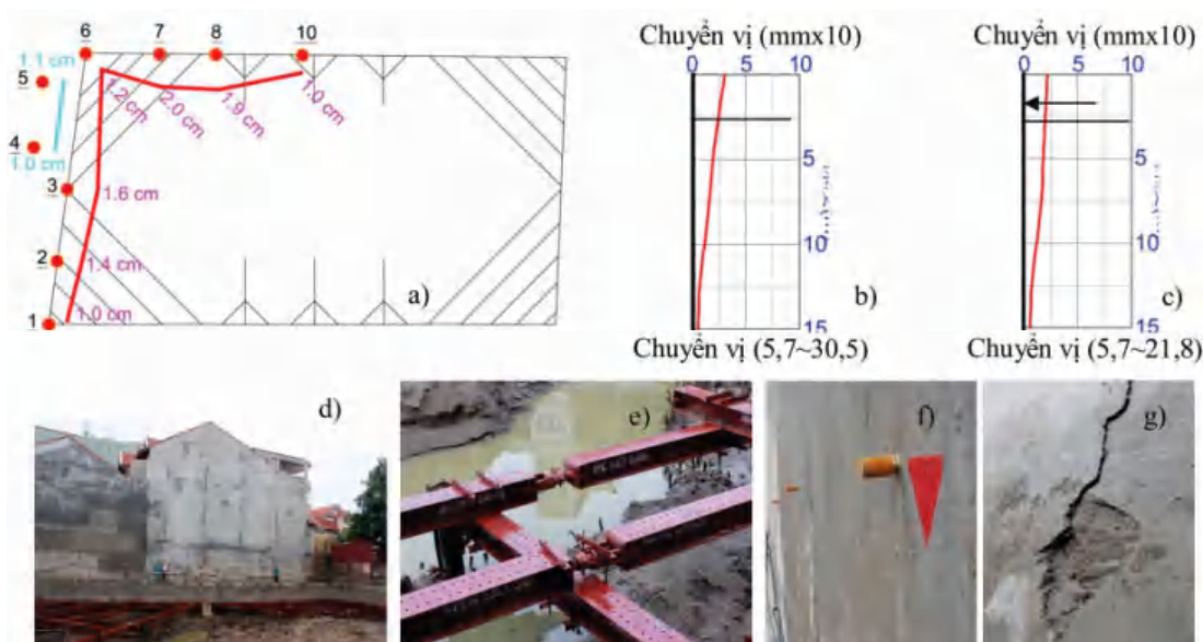
Hình 4: Một số hình ảnh hố móng. a) Văng chống tại vị trí công trình lân cận, b) Chuyển vị của tường khi đào xuống -2,5 m; c) Chuyển vị của tường khi lắp đặt thanh chống -2,0 m; d) Khảo sát tại vị trí công trình lân cận; e) Nước cuốn theo hạt đất mịn và cát vào trong hố móng; f) Bố trí các móc quan trắc trên công trình lân cận, g) Nút công trình lân cận
