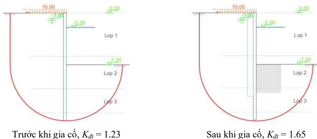
Hình 11: Kết quả tính toán đẩy trôi hố móng
