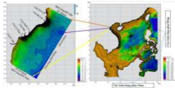
Hình 3: Minh họa lồng ghép dữ liệu biên
