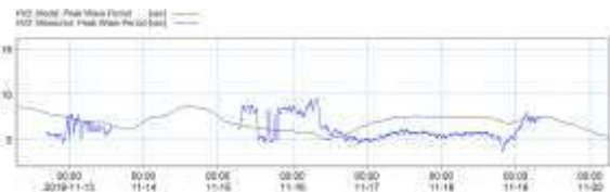
Hình 6: So sánh chu kỳ sóng giữa tính toán mô hình và thực đo
