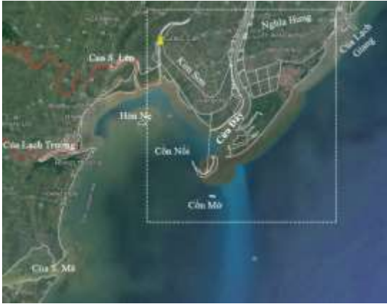
Hình 1: Phạm vi nghiên cứu
