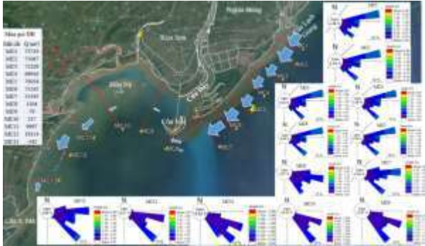
Hình 8: Hoa sóng và dòng vận chuyển dọc bờ trong mùa gió Đông Bắc
