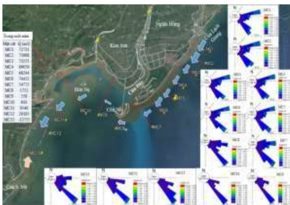
Hình 10: Hoa sóng và dòng vận chuyển dọc bờ trong năm
