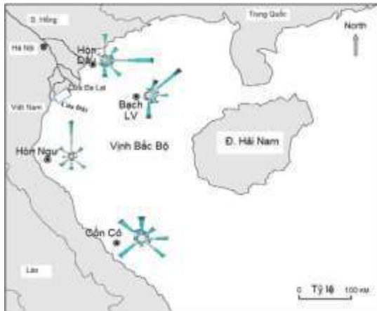
Hình 2: Hoa gió tại các vị trạm xung quanh khu vực nghiên cứu
