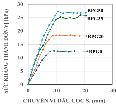
Hình 3.19. Sức kháng thành đơn vị trung bình của các cọc.
