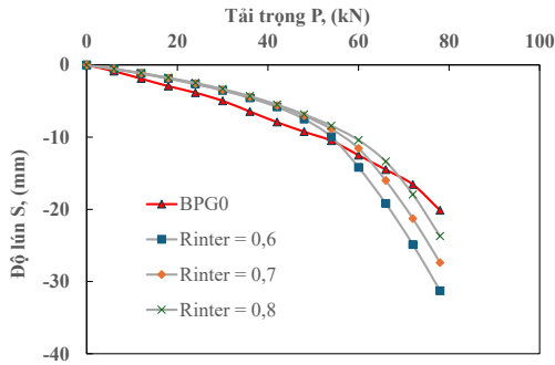
Hình 4.2. So sánh giữa kết quả mô phỏng và thí nghiệm cọc BPG0 khi thay đổi R_{inter} = [0,6 \div 0,8]
