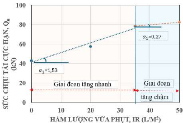
Hình 3.13. Ảnh hưởng hàm lượng vữa phụ đến giá trị sức chịu tải cực hạn của cọc.
