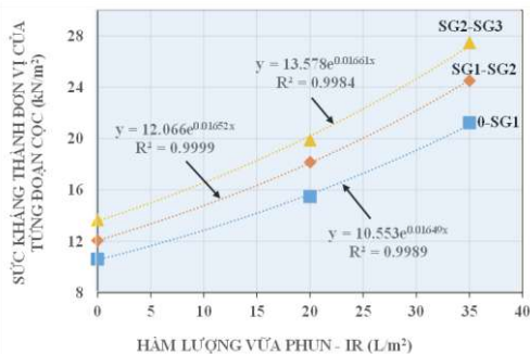
Hình 3.20. Biểu đồ quan hệ giữa sức kháng thành đơn vị và hàm lượng vữa phụt
