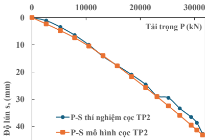
Hình 4.16. So sánh P–S giữa mô phỏng và thí nghiệm của cọc phụt vữa TP2 tại công trình Friendship Tower.
