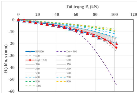
Hình 4.3. Biểu đồ P-S của cọc phụt vữa BPG20 theo đường kính quy đổi thử dần, trường hợp R_{inter} = 0,8
