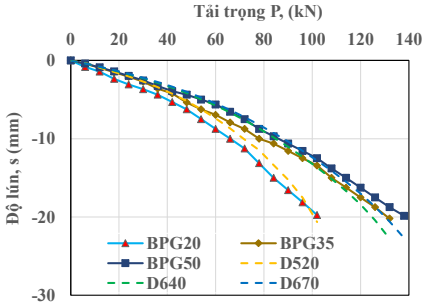
Hình 4.6. Biểu đồ P-S của cọc phụt vữa tương ứng với đường kính qui đổi đã xác định, trường hợp R_{inter} = 0,9
