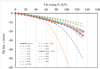
Hình 4.4. Biểu đồ P-S của cọc phụt vữa BPG35 theo đường kính quy đổi thử dần, trường hợp R_{inter} = 0,8
