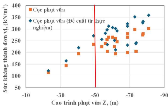
Hình 3.24. Biểu đồ quan hệ giữa giá trị sức kháng thành đơn vị của cọc tính theo công thức (3.2) và kết quả tương ứng từ TN nén tĩnh của 8 công trình khác nhau
