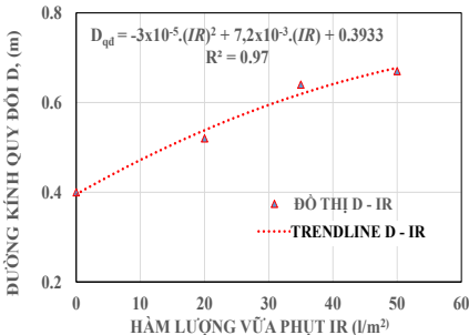
Hình 4.8. Đồ thị quan hệ giữa D_{qd} và IR của cọc phụt vữa xác định bằng phương pháp số
