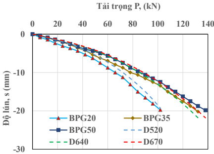
Hình 4.7. Biểu đồ P-S của cọc tương ứng với đường kính qui đổi đã xác định, trường hợp R_{inter} = 1,0
