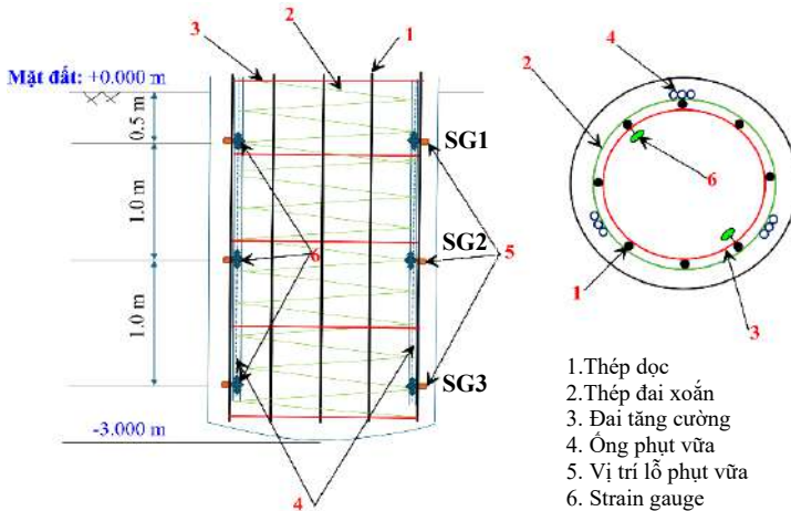
Hình 3.5. Cấu tạo của các cọc thí nghiệm
