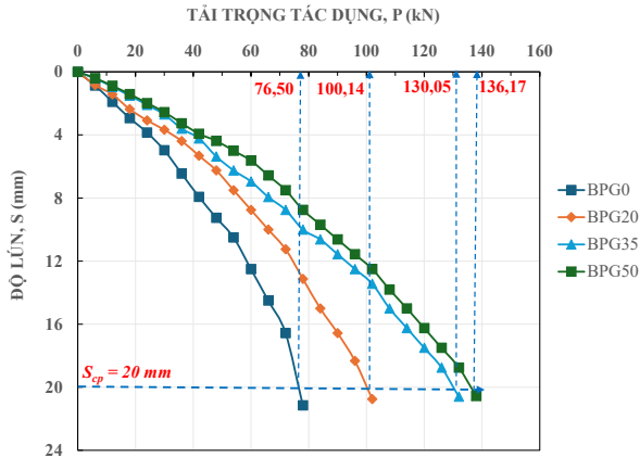
Hình 3.12. Đường cong P -S của các cọc thí nghiệm
