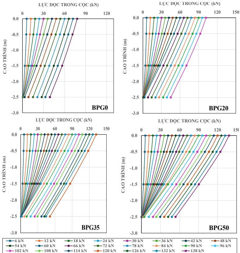
Hình 3.17. Biểu đồ phân bố lực dọc trục của các cọc thí nghiệm
