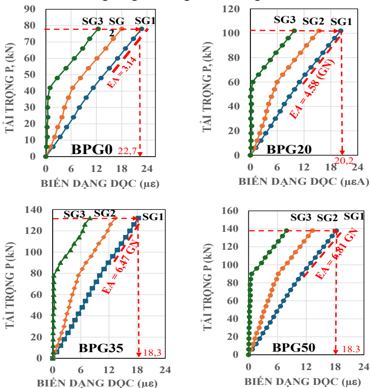
Hình 3.16. Số liệu biến dạng của các cọc BPG0, BPG20, BPG35 và BPG50
