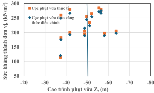
Hình 3.26. Biểu đồ quan hệ giữa giá trị sức kháng thành đơn vị của cọc xác định theo công thức điều chỉnh và kết quả phân tích số liệu của công trình Sông Đà Riverside và Sông Việt.
