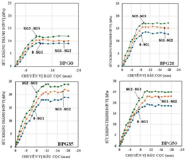
Hình 3.18. Biểu đồ quan hệ giữa sức kháng thành đơn vị và chuyển vị đầu cọc
