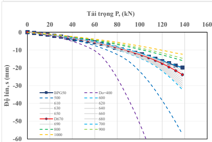
Hình 4.5. Biểu đồ P-S của cọc phụt vữa BPG50 theo đường kính quy đổi thử dần, trường hợp R_{inter} = 0,8
