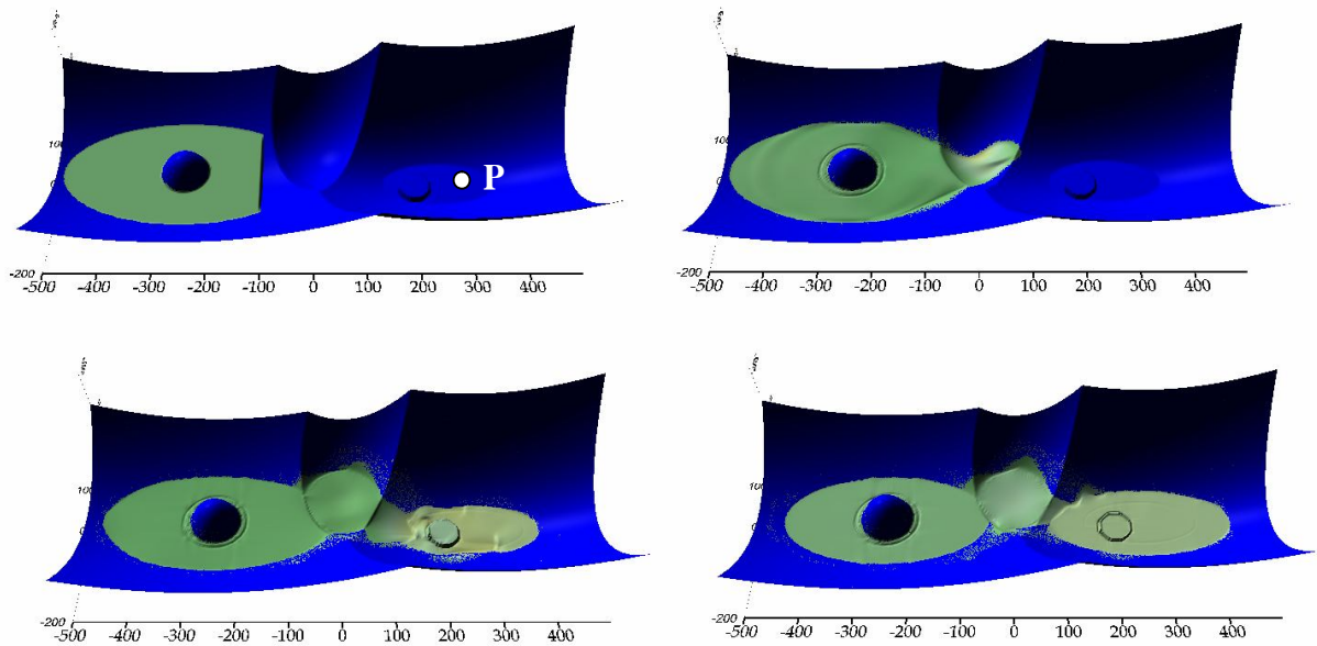
Hình 4: Sự lan truyền sóng gián đoạn trên kênh có địa hình phức tạp tại t = 0s; 10s; 100s và 500s ứng với kích thước lưới \Delta x = \Delta y = 2,5m
