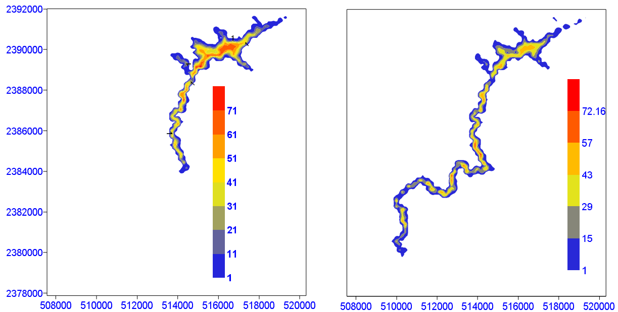
Hình 6: Bản đồ ngập lụt theo tình huống vỡ đập Nậm Chiến lúc t = 500\text{s} và 1500\text{s}
