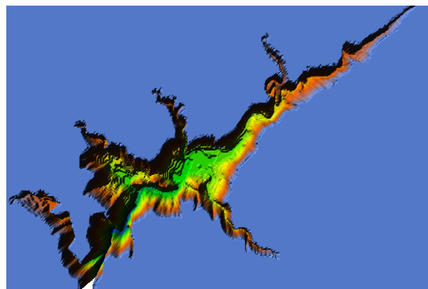
Hình 5: Bản đồ DEM lòng hồ Nậm Chiến
