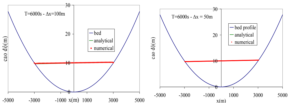
Hình 1: Sự dao động mực nước trong chảo parabol tính với hai loại lưới 100m và 50m
