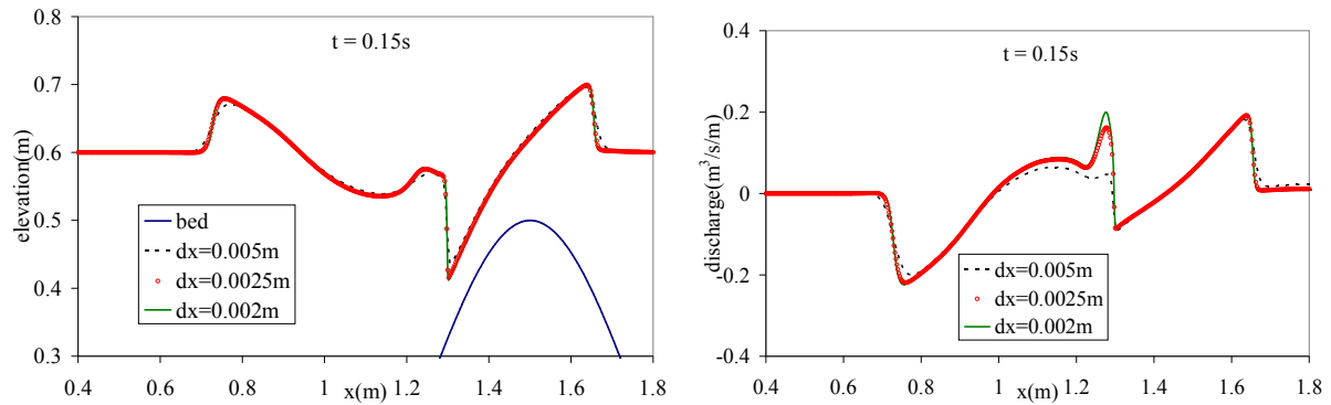
Hình 3: Quá trình mực nước và lưu lượng ứng với \Delta x = 0,005m ; 0,0025m và 0,002m
